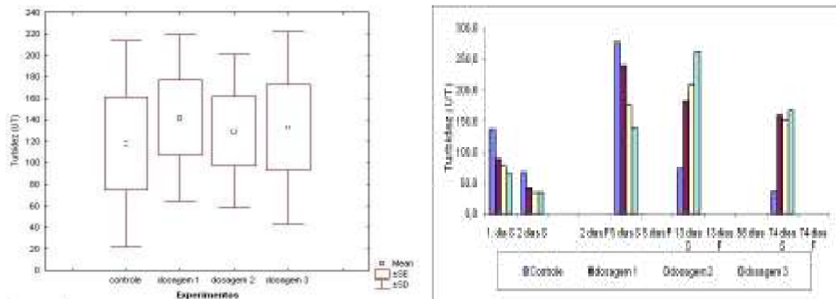
Figura 11: Resultados das análises de turbidez das amostras em todos os contêineres durante o período do experimento.
